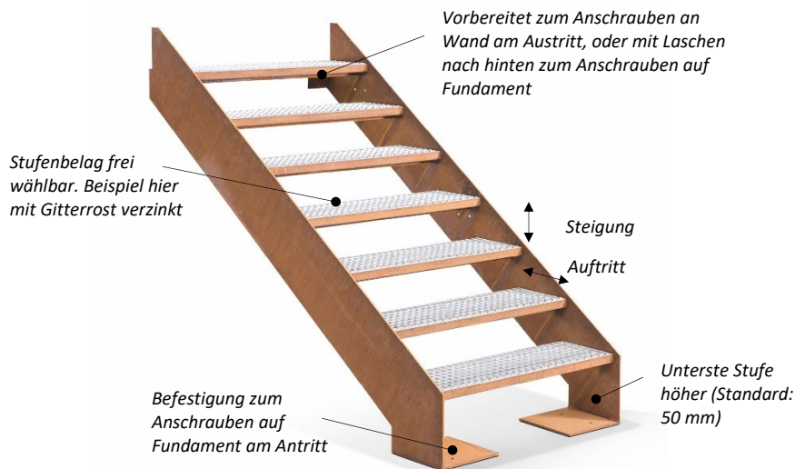
Beispiel Wangentreppe mit Trittstufen aus feuerverzinktem Gitterrost
