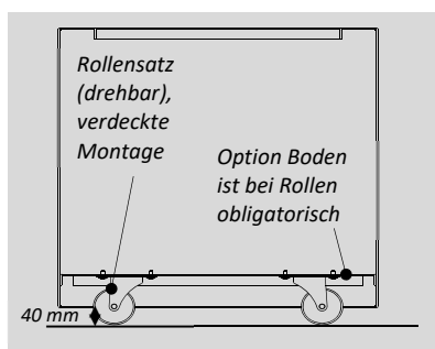
Beispiel Rollensatz mit Pflanzgefäß als Schemazeichnung...
