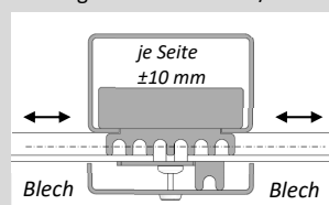
Montagevariante 3: Blech/Blech
