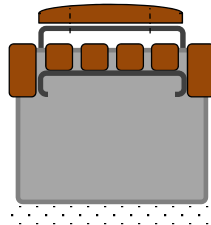
Seitenlehne Typ SL26 Runder Bügel ø48 mm
