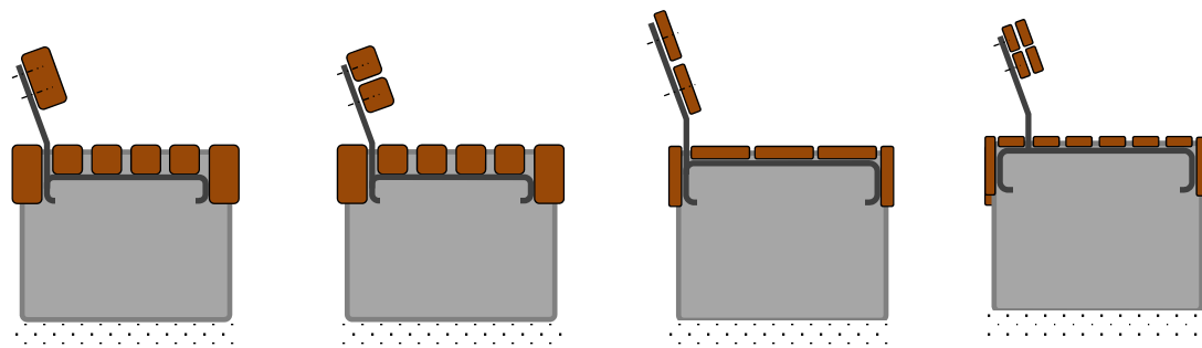
Rückenlehne 100% Hartholz Querschnitt 1x130x65 mm
