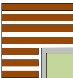
Sitzbankecken-Variante 5: Längs-quer gemischt, lange Seite gerade
