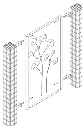
Montage VISTA zwischen Gabionenkörben
