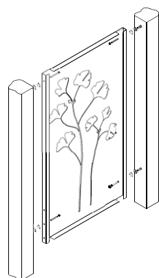
Montage VISTA zwischen zwei Steinsäulen
