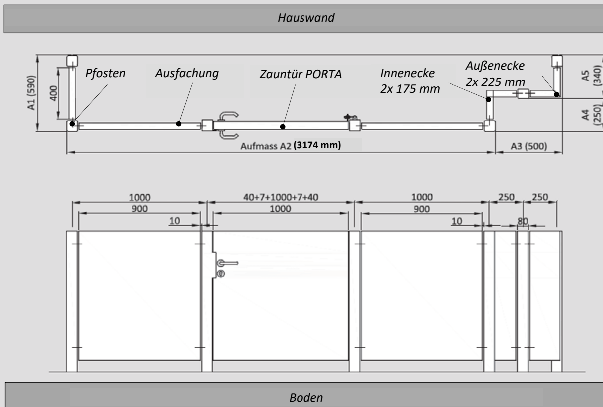
Beispiel Abmessungen für Aufmaß Zaunsystem MIAMI für Ausfachung
