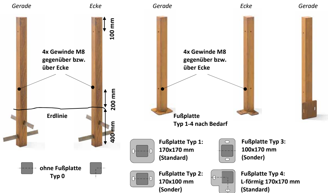
Befestigung Zaunpfosten MIAMI zum Einbetonieren
