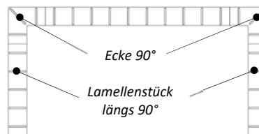
Aufbau Lamellenzaun 90°
