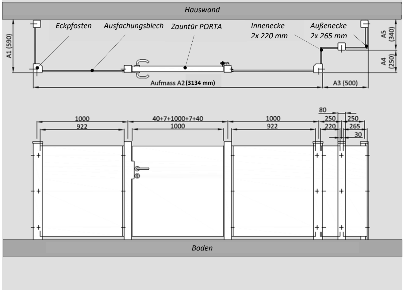
Beispiel Abmessungen für Aufmaß Zaunsystem BOSTON für Ausfachung
