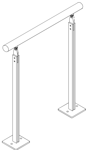
Edelstahlhandlauf \varnothing 40 mm mit Flachpfosten Querschnitt 2 \times 40 \times 10 mm 2 mit Grundplatte 120 \times 120 mm 2
