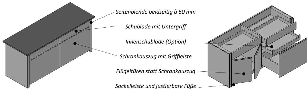
Unterschrank mit Schrankauszug und Schubladen (Darstellung mit Arbeitsplatte)
